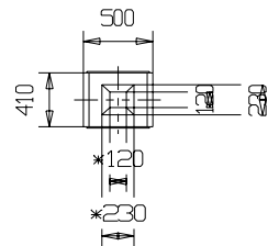
Draufsicht Füllstation
