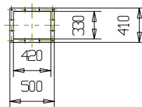
Anschlußflansch Kopfabgabe
