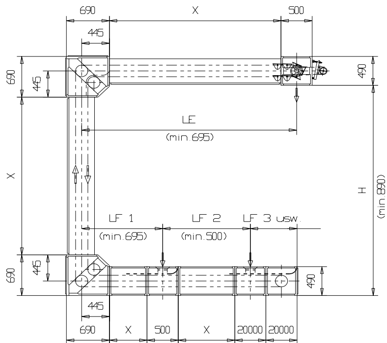
Draufsicht Füllstation
