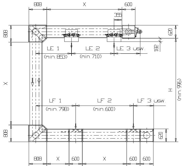
Draufsicht Füllstation
