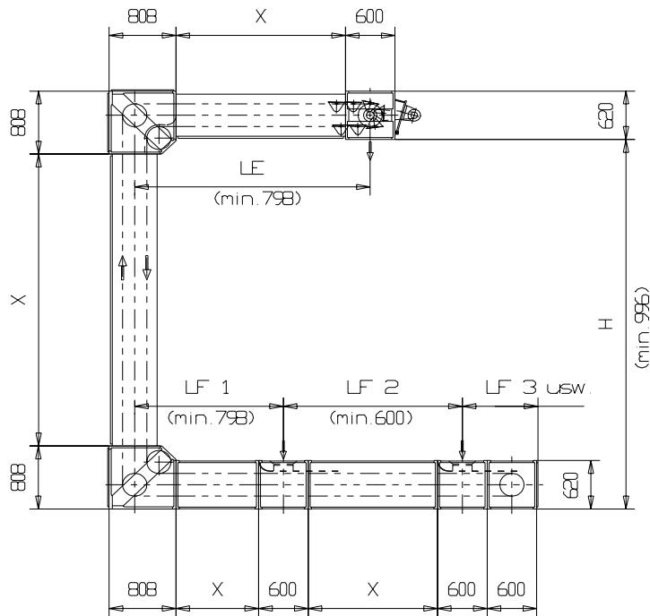
Draufsicht Füllstation
