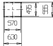
Anschlußflansch Abgabestutzen
