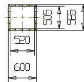
Anschlußflansch Kopfabgabe
