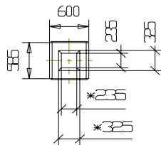
Draufsicht Füllstation
